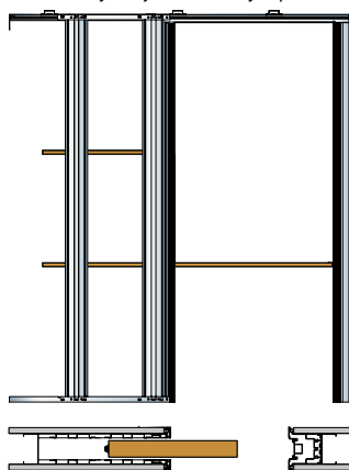
Vodorovný rez jednokrídlovým puzdrom
